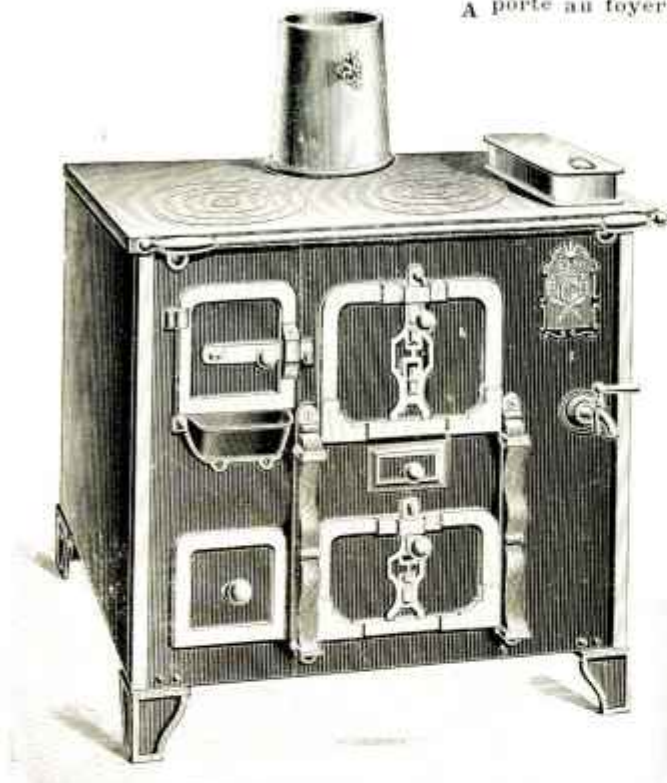
Les numéros 2421 à 2440 sont à foyer très profond spécial pour le bois en grandes bûches
